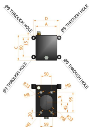
Type 1L – 2L – 3L
